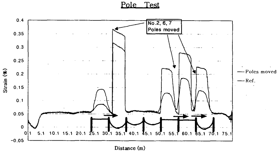
그림 4-6 말뚝 시험 계측 결과
