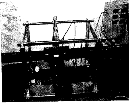
그림 4-1 PVC 파이프 시험
