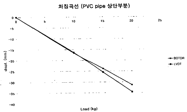
그림 4-4 측정 센서 비교
