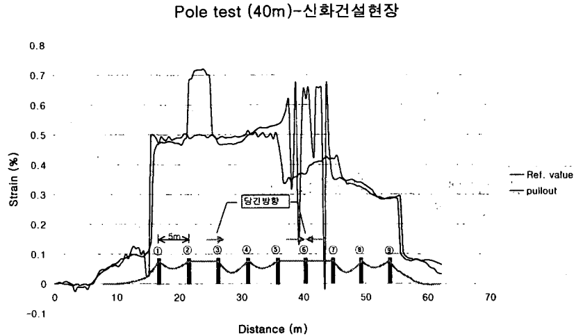
그림 4-9 말뚝시험Ⅱ 계측 결과
