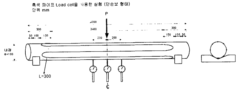
그림 4-2 PVC 파이프 광케이블 부착 위치
