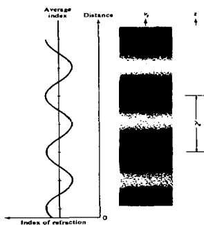
그림 2-1 sound wave와 굴절율 변화
