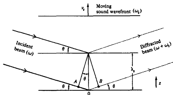
그림 2-2 브래그 조건을 만족하는 광파의 회절
