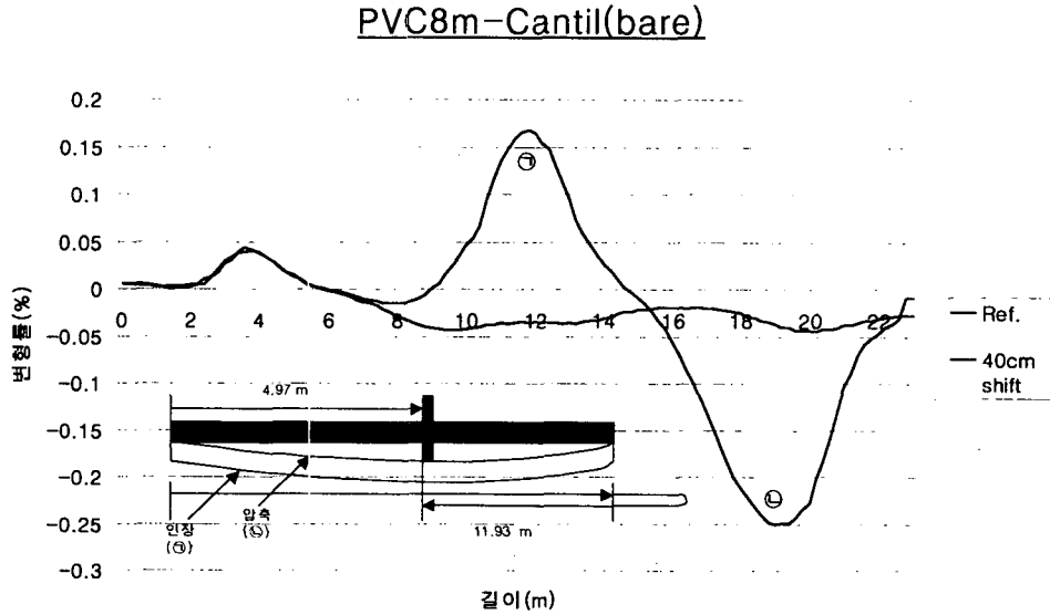
그림 4-12 산란파를 이용한 광센서(BOTDR) 계측 결과
