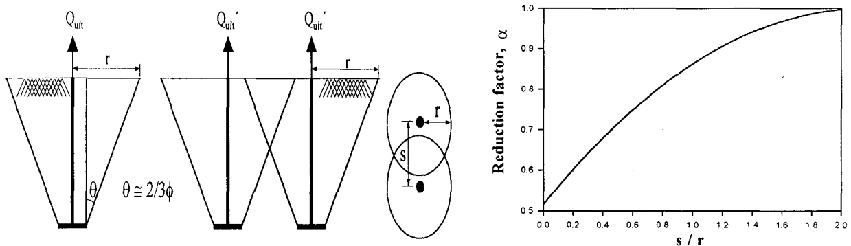
그림 2. 무리효과를 고려한 앵커의 극한인발저항력 감소율(日本土質工學會, 1990)
