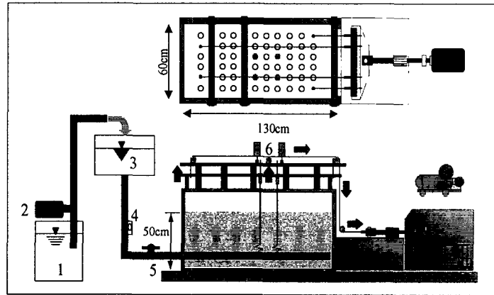
1.저수조 2.양수모터 3.급수조 4.유속계 5.유량조절밸브 6.LVDT 그림 4. 앵커인발시험기 개요도
