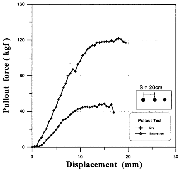
그림 8. 하중-인발변위 관계곡선 (S/B = 4)
