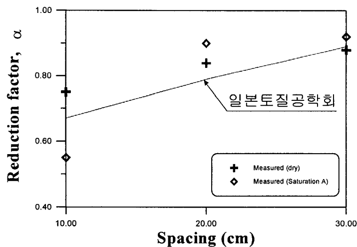
그림 10. 무리앵커의 설치간격에 따른 극한인발저항력 감소율 비교
