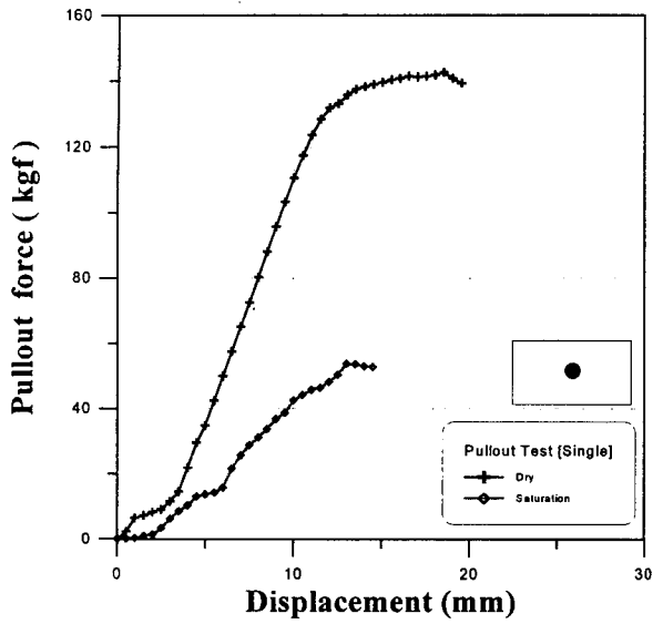
그림 6. 하중-인발변위 관계곡선 (단일 앵커)
