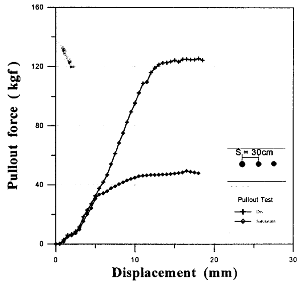
그림 9. 하중-인발변위 관계곡선 (S/B = 6)
