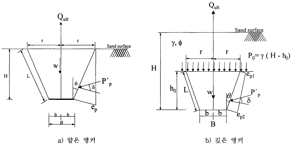
그림 1. 얇은 앵커와 깊은 앵커의 파괴면
