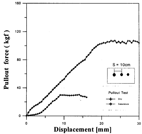
그림 7. 하중-인발변위 관계곡선 (S/B=2)
