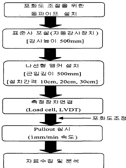
그림 5. 실험순서도
