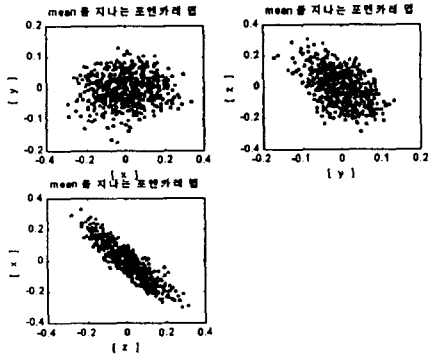
그림 5. 진동 신호의 포엔카레 단면
