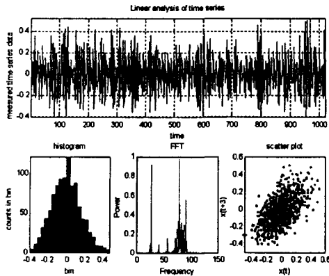
그림 1. 베어링 진동신호의 시계열과 히스토그램, FFT, 재구성한 어트랙터
