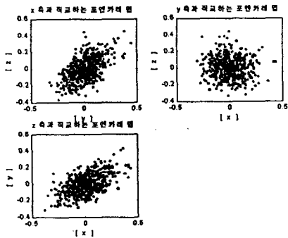
그림 6. 진동신호의 포엔카레 단면
