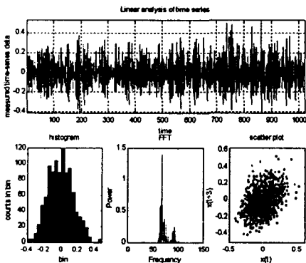
그림 2. 베어링 진동신호의 시계열과 히스토그램, FFT, 재구성한 어트랙터
