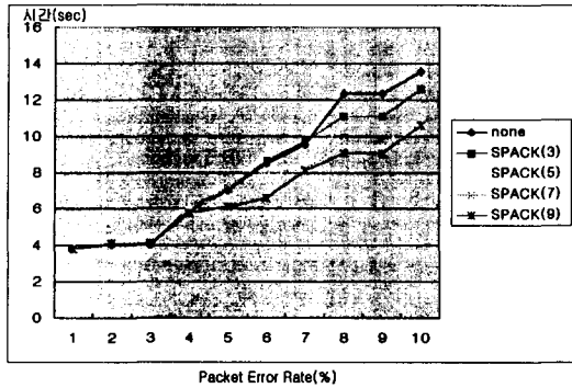
그림 6. 패킷손실율 vs. 전송시간(MSS=1000B)
