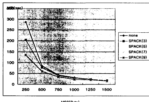
그림 11. MSS vs. 전송시간(500KB전송)
