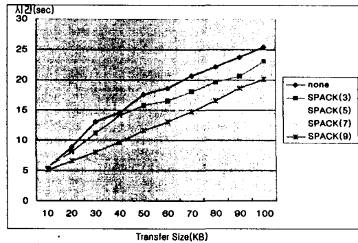
그림 9. 데이터크기 vs. 전송시간(10%손실)
