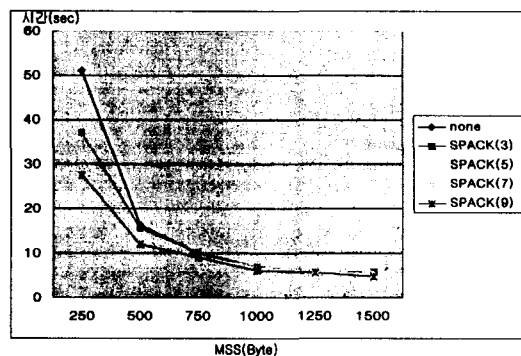
그림 10. MSS vs. 전송시간(100KB전송)
