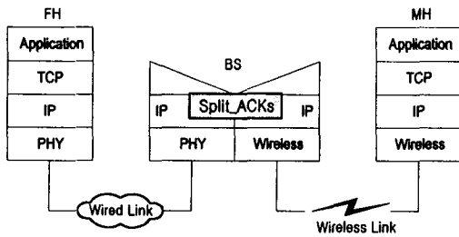
그림 4. Split ACKs 기법의 프로토콜 구조
