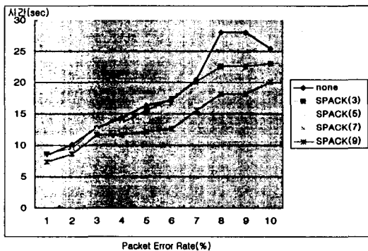
그림 7. 패킷손실율 vs. 전송시간(MSS=500B)
