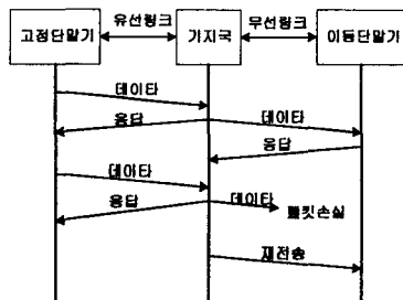
그림 2. I-TCP의 동작원리
