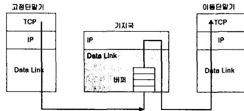
그림 3. Snoop 모듈의 동작원리
