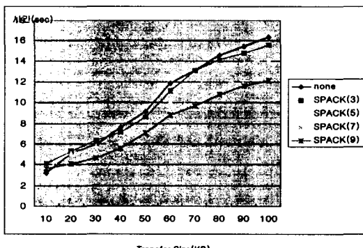
그림 8. 데이터크기 vs. 전송시간(5%손실)
