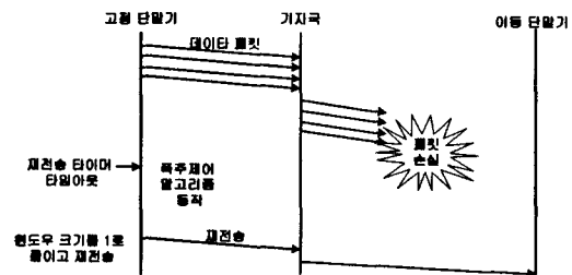
그림 1. 무선통신 환경에서 TCP의 동작
