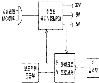
그림1. 기존의 대기전력 차단원리.
