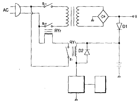
그림3. 대기전력 차단회로
