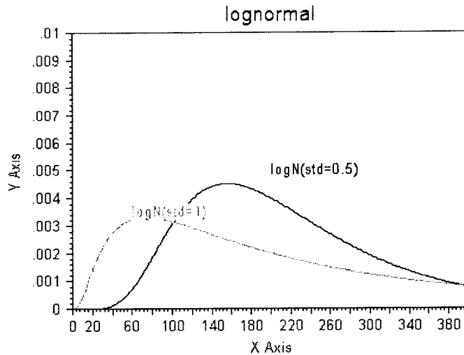
그림 2. 예제1) 데이터에 의한 대수정규분포의 확률밀도 함수
