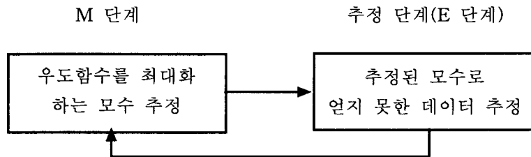
< 그림 3. EM 알고리즘 >
