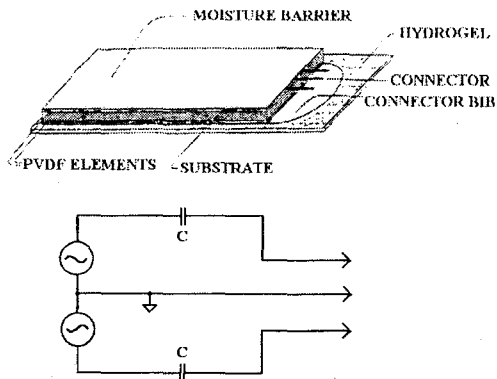
그림 1. PADS 외형과 등가회로(Illustration of the PADS and it's equivalent circuit)
