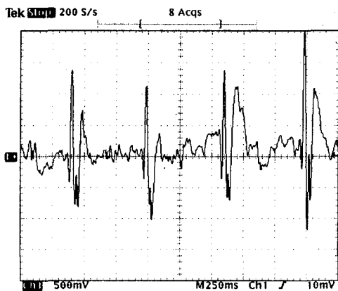
그림 3. Instrumentation amplifier의 출력신호 (A output signal of a instrumentation amplifier)
