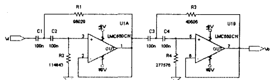
그림 5. Butterworth high-pass filter
