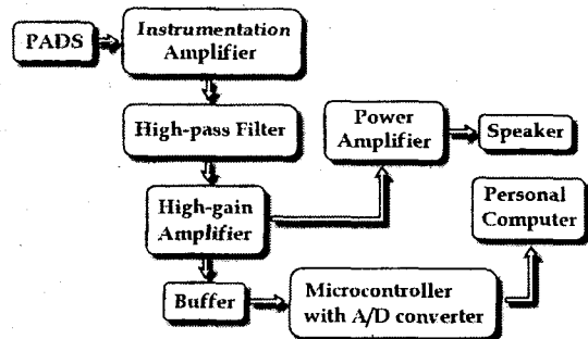
그림 2. 전자 청진 시스템의 전체 블록 다이어그램(The block diagram for a electronic auscultation system)
