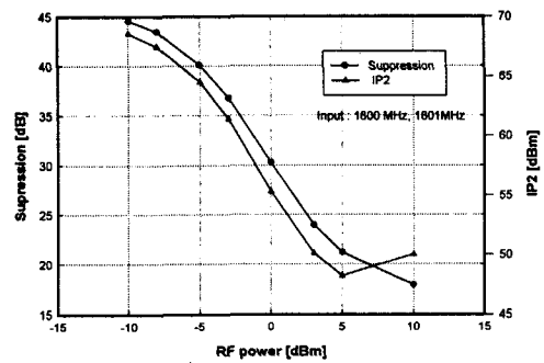
그림5. APDP의 even suppression 특성 측정치.
