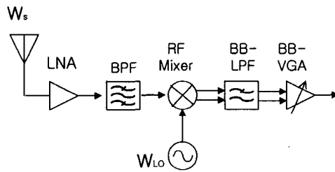
그림4. 헤테로다인 수신기
