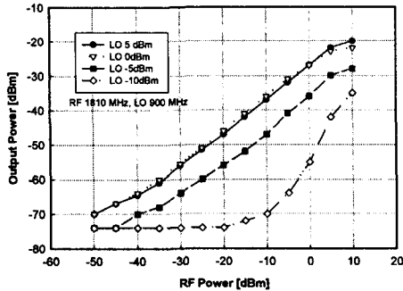
그림3. LO power변화에 대한 응답특성.
