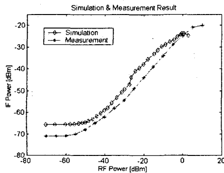
그림6. APDP의 RF power 수신특성 (LO: 900MHz 0dBm, RF: 1815MHz, IF: 15MHz)
