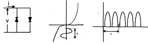
그림1. APDP(Anti Parallel Diode Pair)
