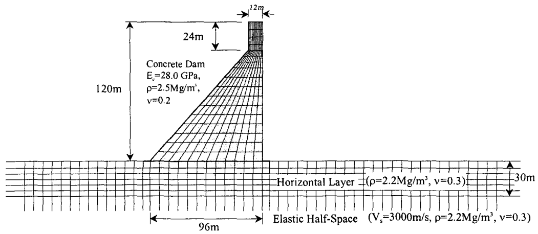
(a) 담수전 댐 구조물 및 유한요소와 무한요소 체는
