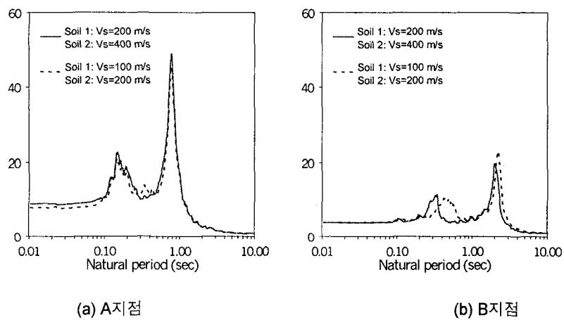
그림 3. 지반조건에 따른 사용후 핵연료 저장구조물의 내부 및 외부 벽체 상단에서의 가속도응답스펙트럼 비교 (5% 감쇠비)
