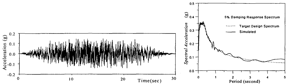
그림 2. 해석에 사용된 입력가속도의 시간이력 및 응답스펙트럼 (PGA=0.14g)
