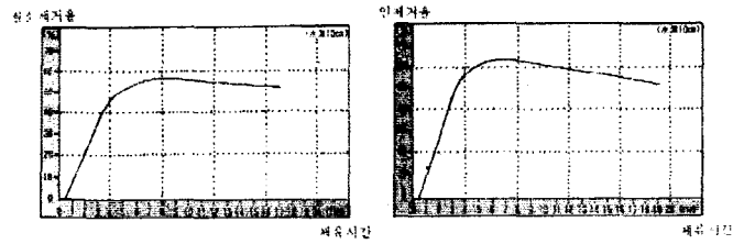
그림 2.1 체류시간과 질소, 인의 제거율 관계
