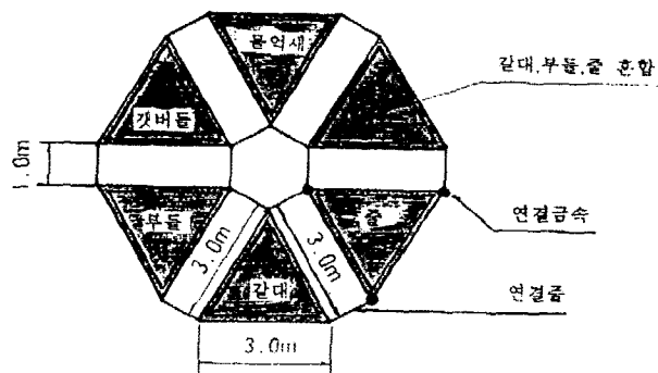
그림 4.2 인공식물섬 설치 (평면도)
