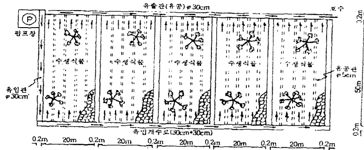
(a) 평면도
