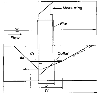
그림 3.2 모형교각 개념도
