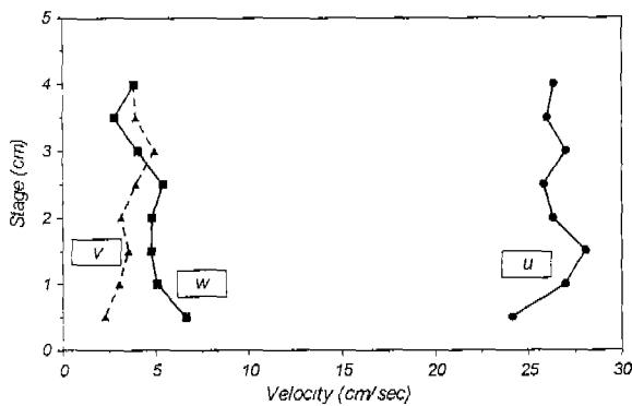
그림 4.1 교각 직상류의 유속분포
