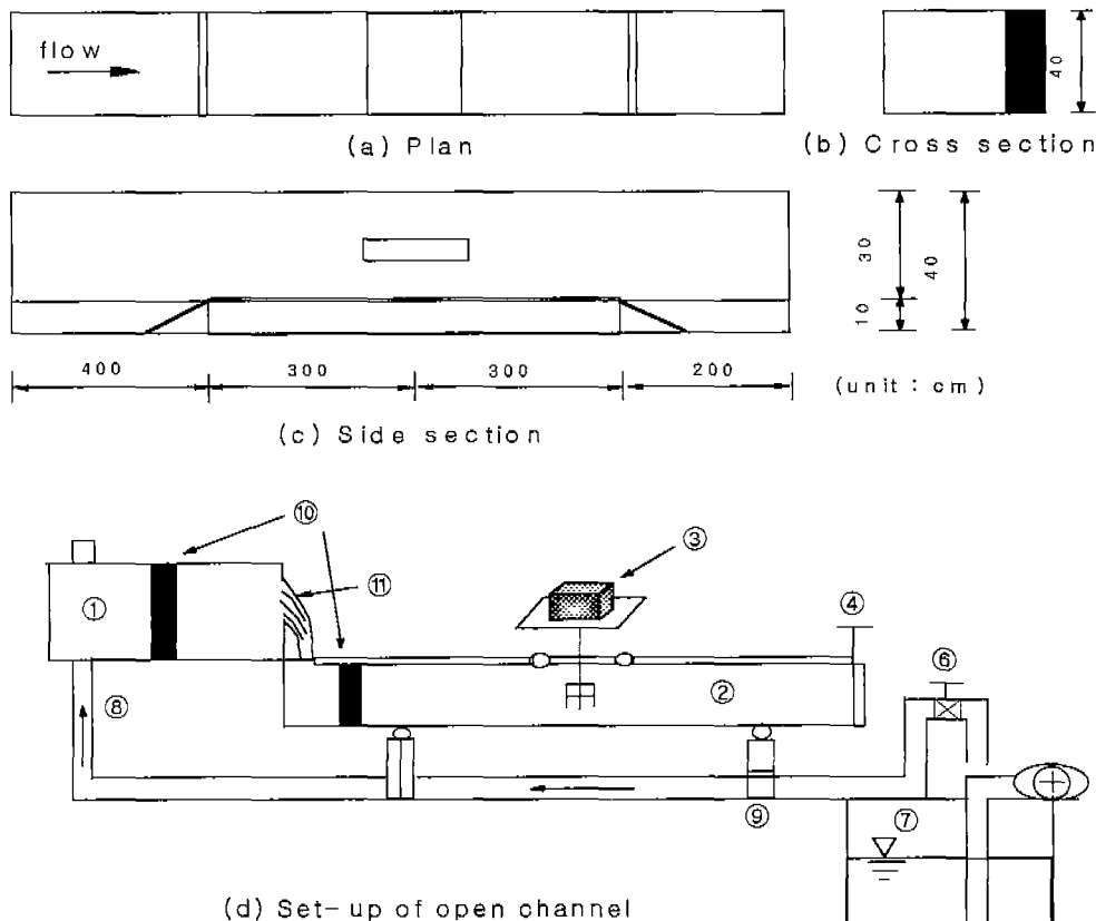
그림 1. 수리모형 실험장치
