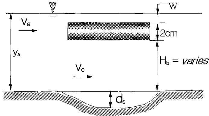
그림 2. 교량상판실험의 구성
