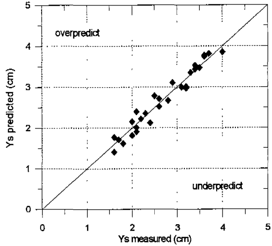
그림 4. 실측세굴심과 예측세굴심의 비교
