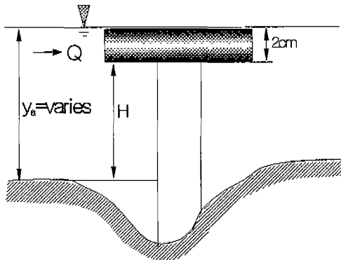
그림 5. 압력흐름실험 구성
