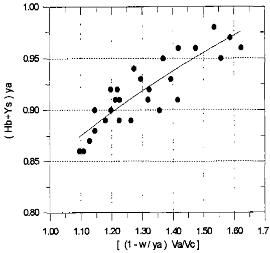
그림 3. 회귀분석결과
