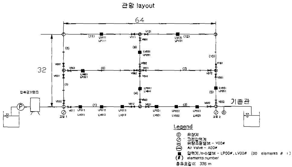
그림 1. 수리모형 layout
