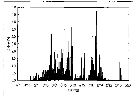
그림 2. 양수장 일별 급수패턴(1995년)
