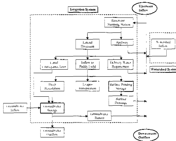
그림 1. REFLOW모형의 계산흐름도
