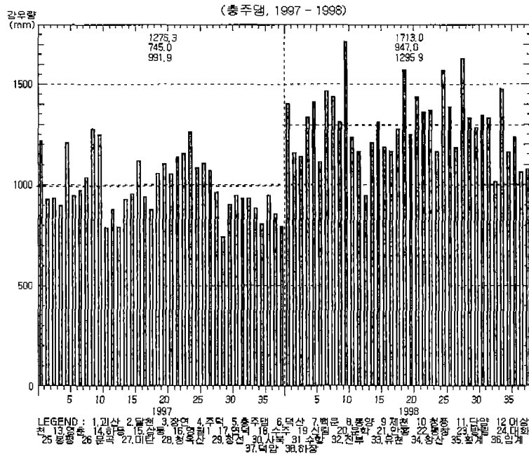
그림 1 충주댐의 연 강수량 분포 예(1997-1998)
