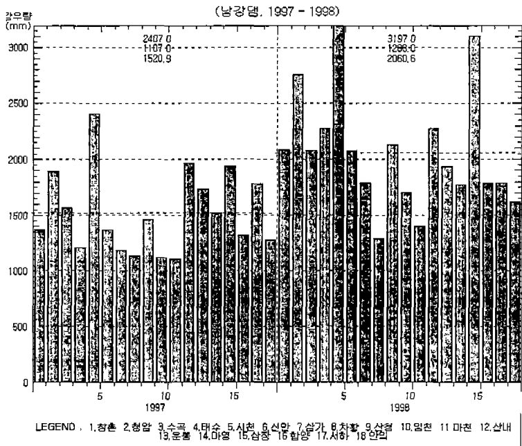
그림 2 남강댐의 연 강수량 분포 예(1997-1998)
