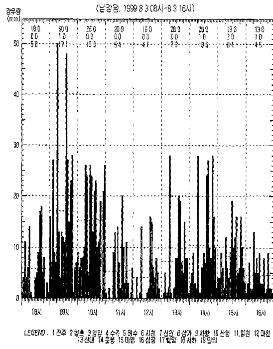
그림 6 남강댐의 시간 강우량 공간분포 예(1999.8.3.8-16시)
