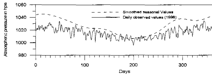
그림 4 소양강댐 유역의 기압 관측자료 (1998, 일단위) & seasonal values
