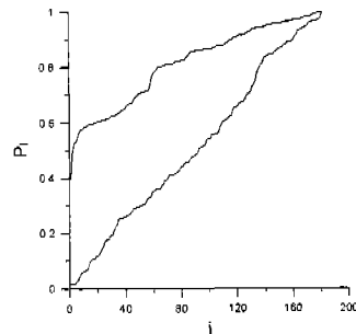
그림 1 Periodogram(강우)
