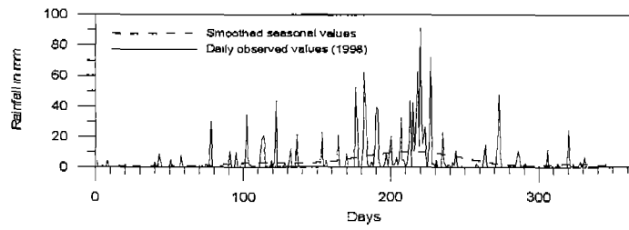
그림 3 소양강댐 유역의 강우 관측자료 (1998, 일단위) & seasonal values
