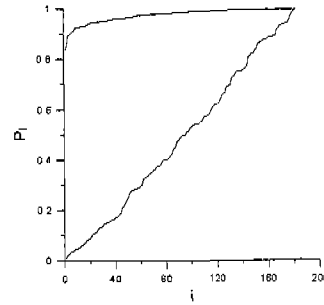
그림 2 Periodogram(기압)
