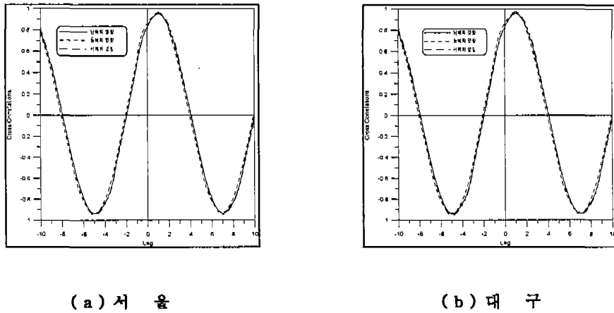
(a) 서울 (b) 대구 그림 2 각 도시의 기온과 해역별 해수면 온도와의 상관관계 (입력자료계열:해양수온, 출력자료계열:각 도시별 기온)
