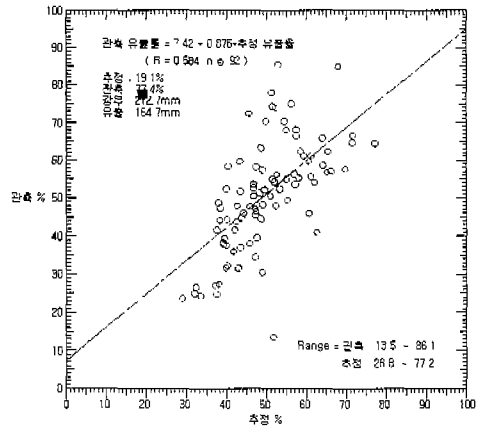
그림 10 낙동강수계(1998.10.1-3.31, 신안)
