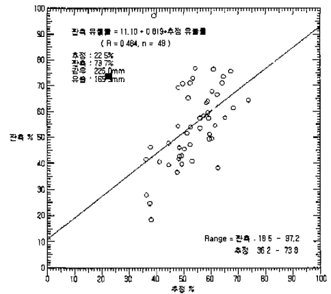
그림 18 섬진/영산강(1998.10.1-3.31,쌍치)
