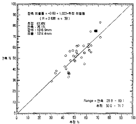
그림 13 금강 수계(1998.1.1-12.31, 수통)
