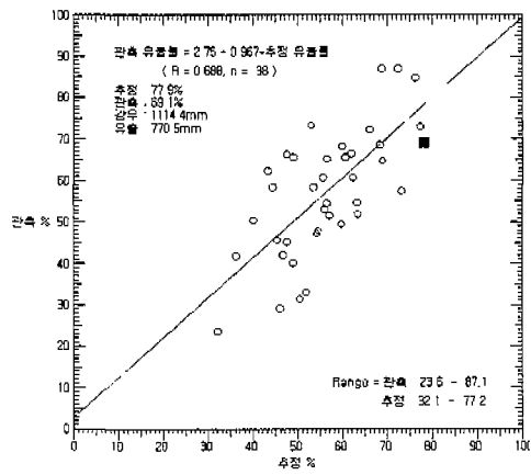
그림 16 금강 수계(1998.6.21-9.30, 수통)
