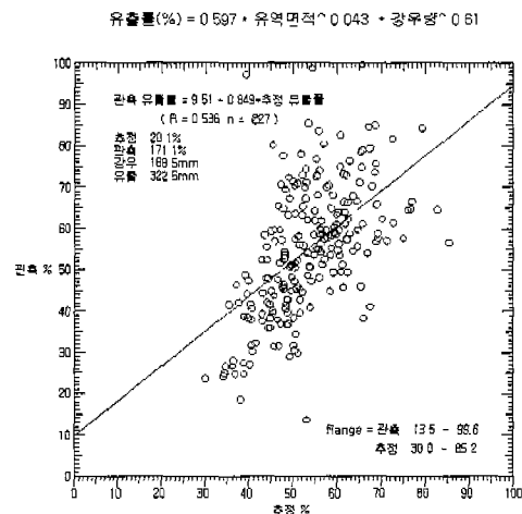
그림 2 전 수계(1998.10.1-3.31, 호탄)
