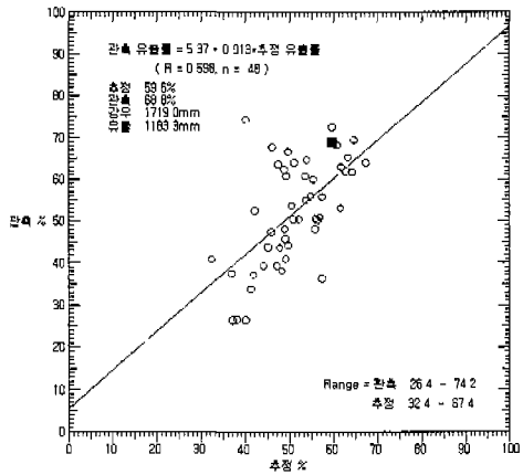
그림 17 섬진/영산강(1998.1.1-12.31,쌍치)
