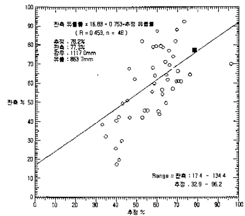
그림 20 섬진/영산강(1998.6.21-9.30,쌍치)
