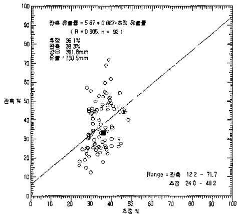
그림 11 낙동강 수계(1998.4.1-6.20, 신안)
