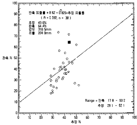
그림 15 금강 수계(1998.4.1-6.20, 수통)
