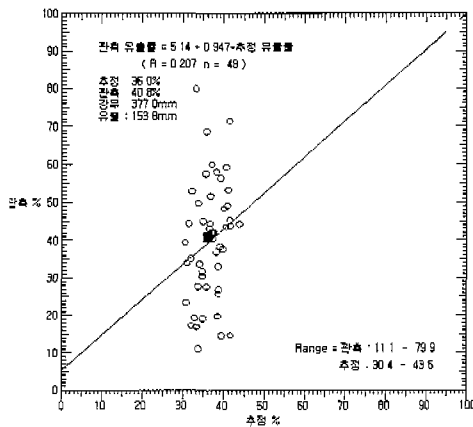
그림 19 섬진/영산강(1998.4.1-6.20,쌍치)
