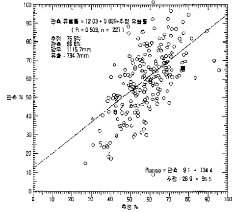
그림 4 전 수계(1998.6.21-9.30, 호탄)
