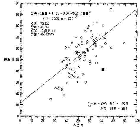
그림 12 낙동강수계(1998.6.21-9.30, 신안)
