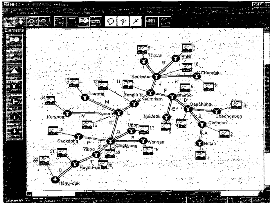
그림 2 HEC-HMS의 GUI를 이용한 금강유역의 Subbasin Model
