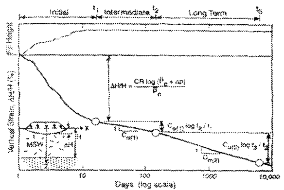
그림 2. 폐기물 매립지반의 침하 모델 (Stulis et al. 1995)
