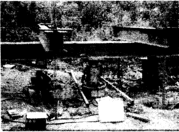
그림 5. 정재하시험
