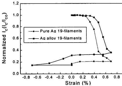
2) 19 filaments Bi-2223/Ag tapes
