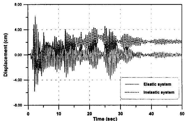
그림 5. 단자유도계의 탄성 및 비탄성 거동
