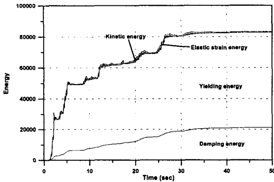
그림 8. 비탄성 시스템의 에너지 시간이력
