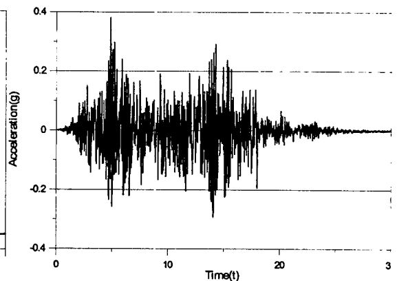
그림 3. 인공지진의 가속도 시간이력(0.154g)
