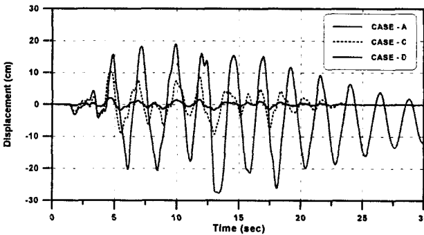
그림 11. 10층 건축물 5층 변위의 시간이력
