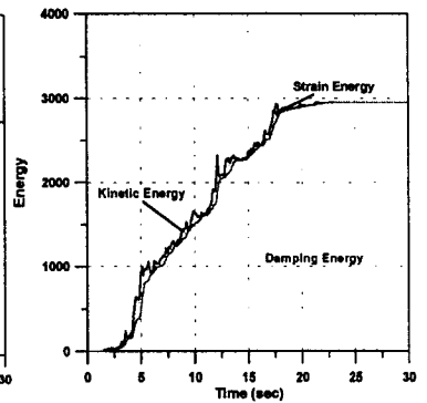
그림 20. Case D의 에너지 시간이력
