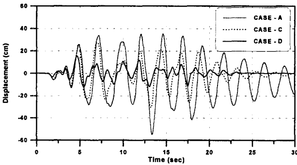
그림 10. 10층 건축물 최상층 변위의 시간이력
