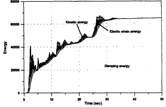
그림 7. 탄성시스템의 에너지 시간이력
