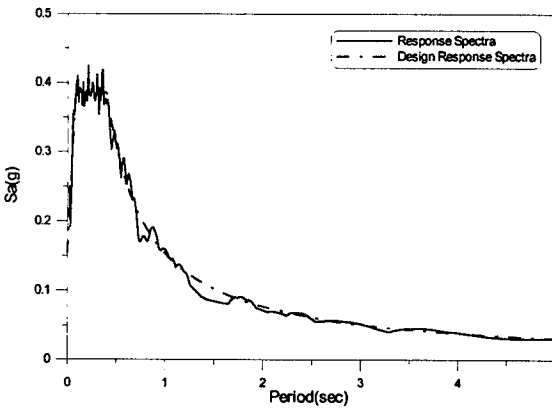
그림 2. 인공지진의 응답스펙트럼(0.154g)
