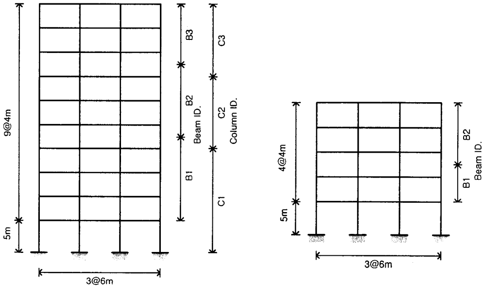
그림 1. 해석 모델
