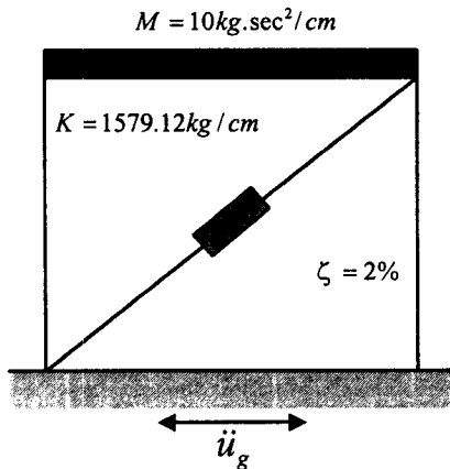
그림 4. 단자유도계 시스템
