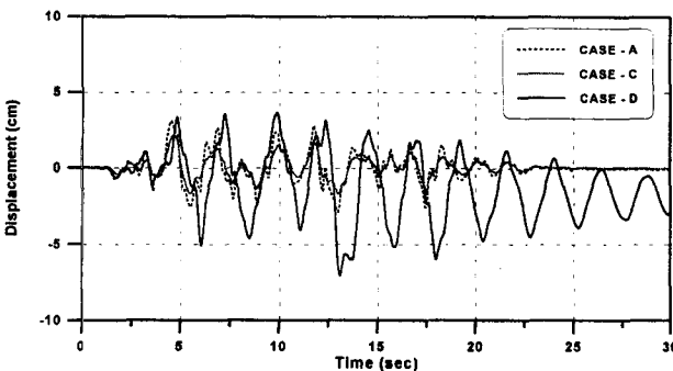
그림 12. 10층 건물 2층 변위의 시간이력
