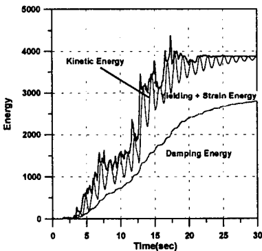
그림 18. Case A의 에너지 시간이력
