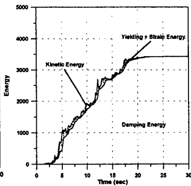
그림 19. Case C의 에너지 시간이력
