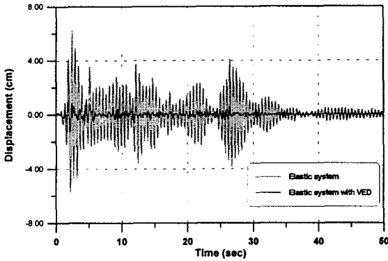
그림 6. 감쇠기가 설치된 시스템의 거동
