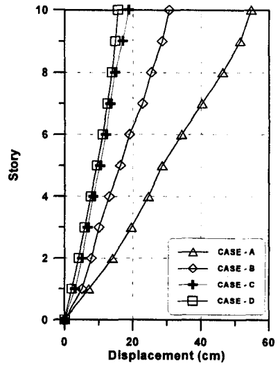
그림 13. 각 층 최대 변위
