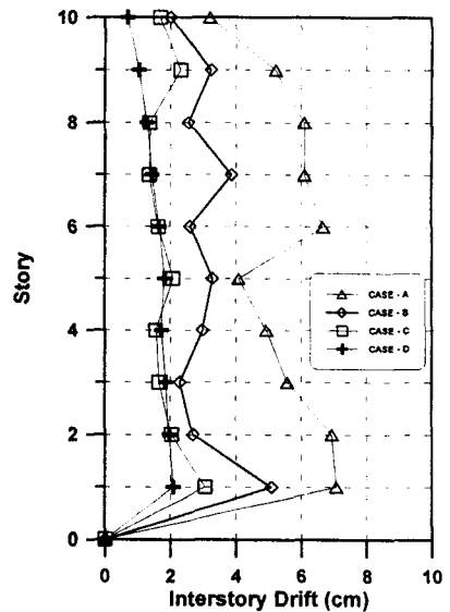
그림 14. 최대 층간 변위
