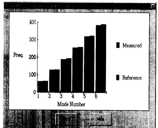
그림 12. 손상 및 비손상 구조의 고유진동수
