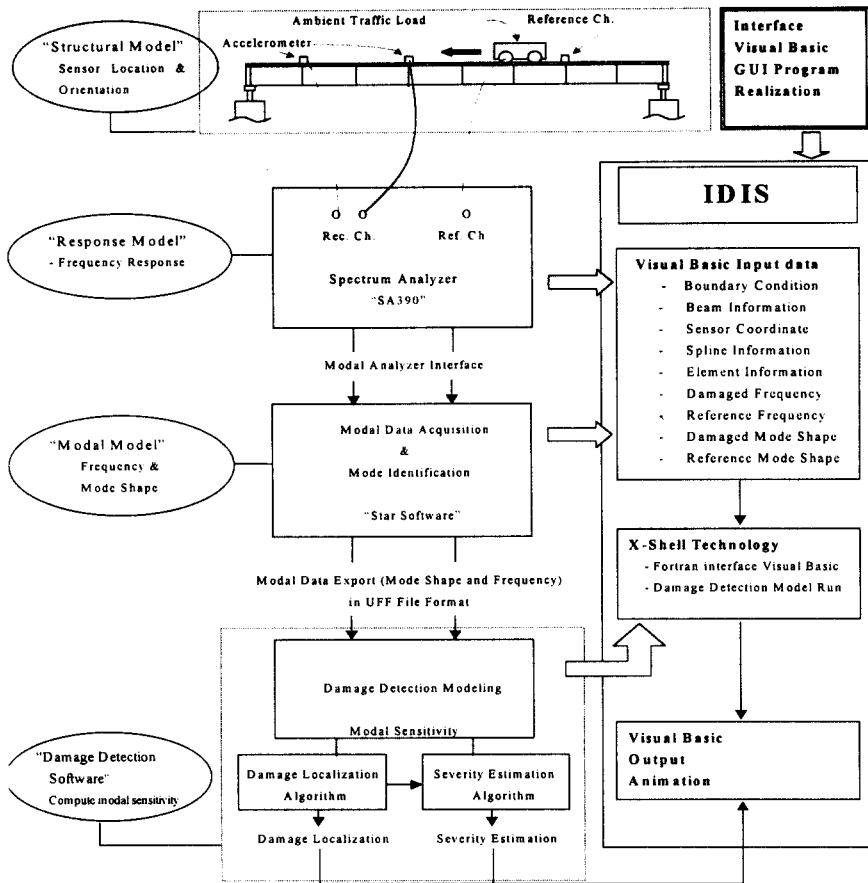
그림 3. 손상검색 자동화체계 계통도
