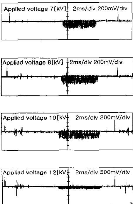
그림 4 연면방전의 방전전류 파형 Fig. 4 Current waveform of surface discharge
