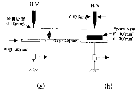
그림 1 전극구성도
