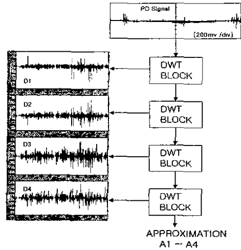
그림 2 이산웨이블릿 변환
