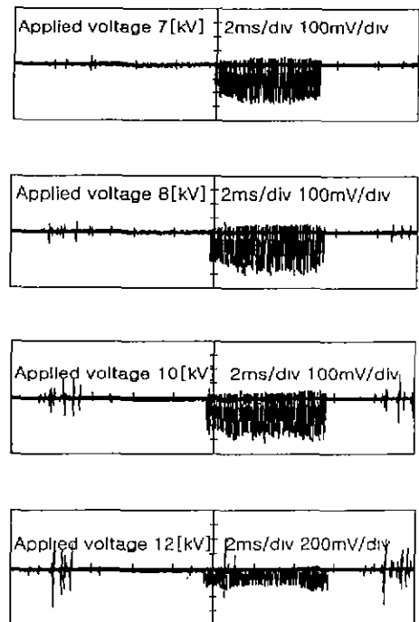
그림 3 코로나방전의 방전전류 파형
