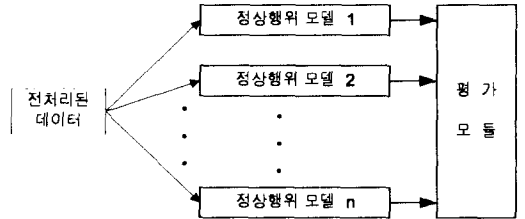
그림 2. 정상행위 모델링
