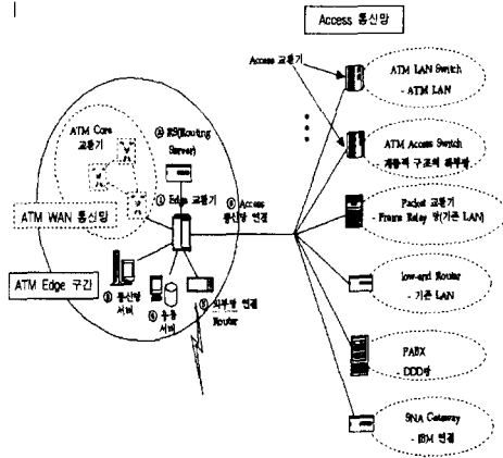
<그림 3> ATM Edge 구간 설계 모델
