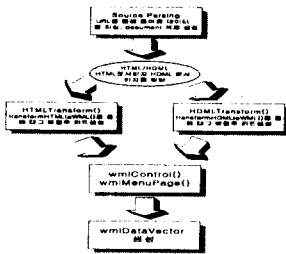
[그림 3] 시스템 내부 구조
