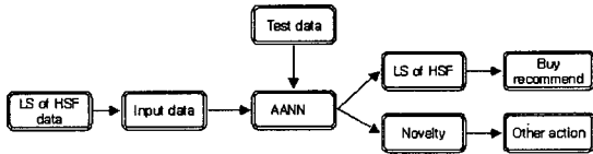
그림 2. 시스템 구조
