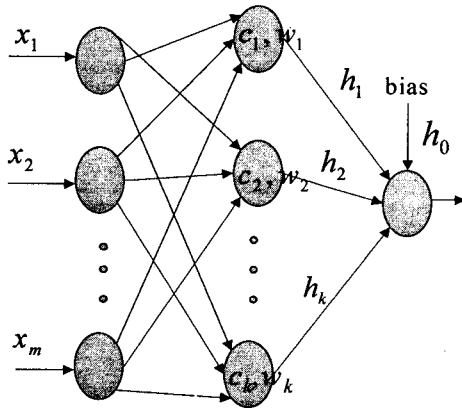
그림 1 : RBF 신경망의 일반적인 구조
