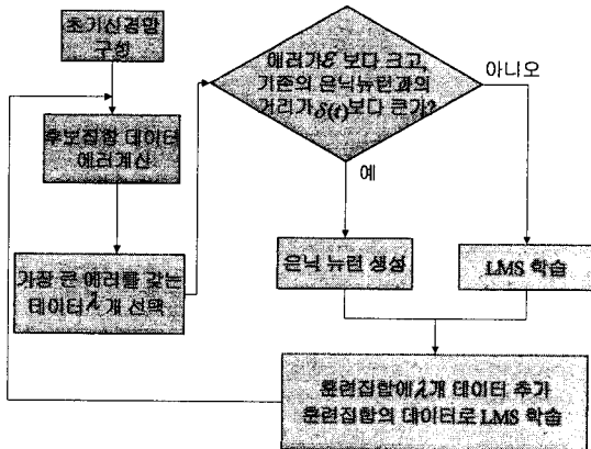
그림 2 : ARAN의 알고리즘
