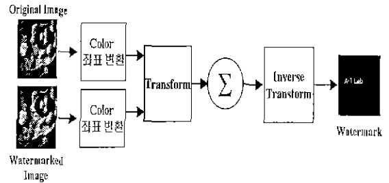
[그림 1] Watermark 삽입 알고리즘
