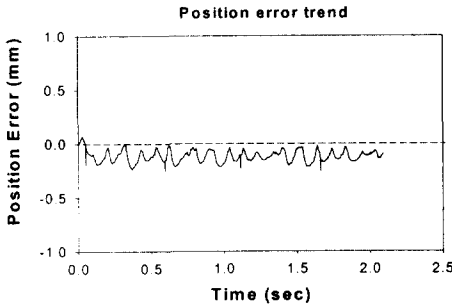
Fig. 3 Position error(Medium)
