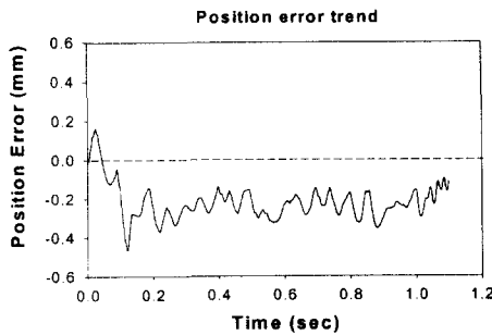
Fig. 4 Position error(Fast)
