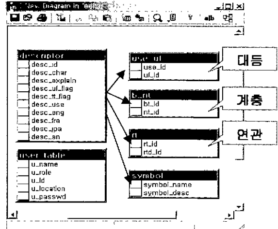
[그림 2] 데이터베이스에 저장된 시소러스 구조
