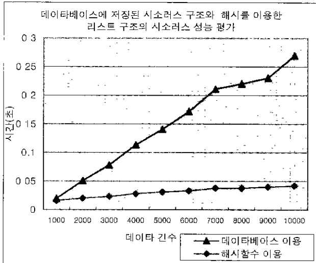
[그림 7] 데이터베이스에 저장된 시소러스 구조와 해시를 이용한 리스트 구조의 성능 평가 결과
