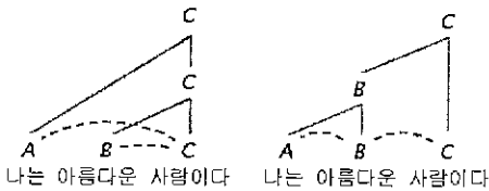
그림 4 CNF-의존문법에 의한 분석
