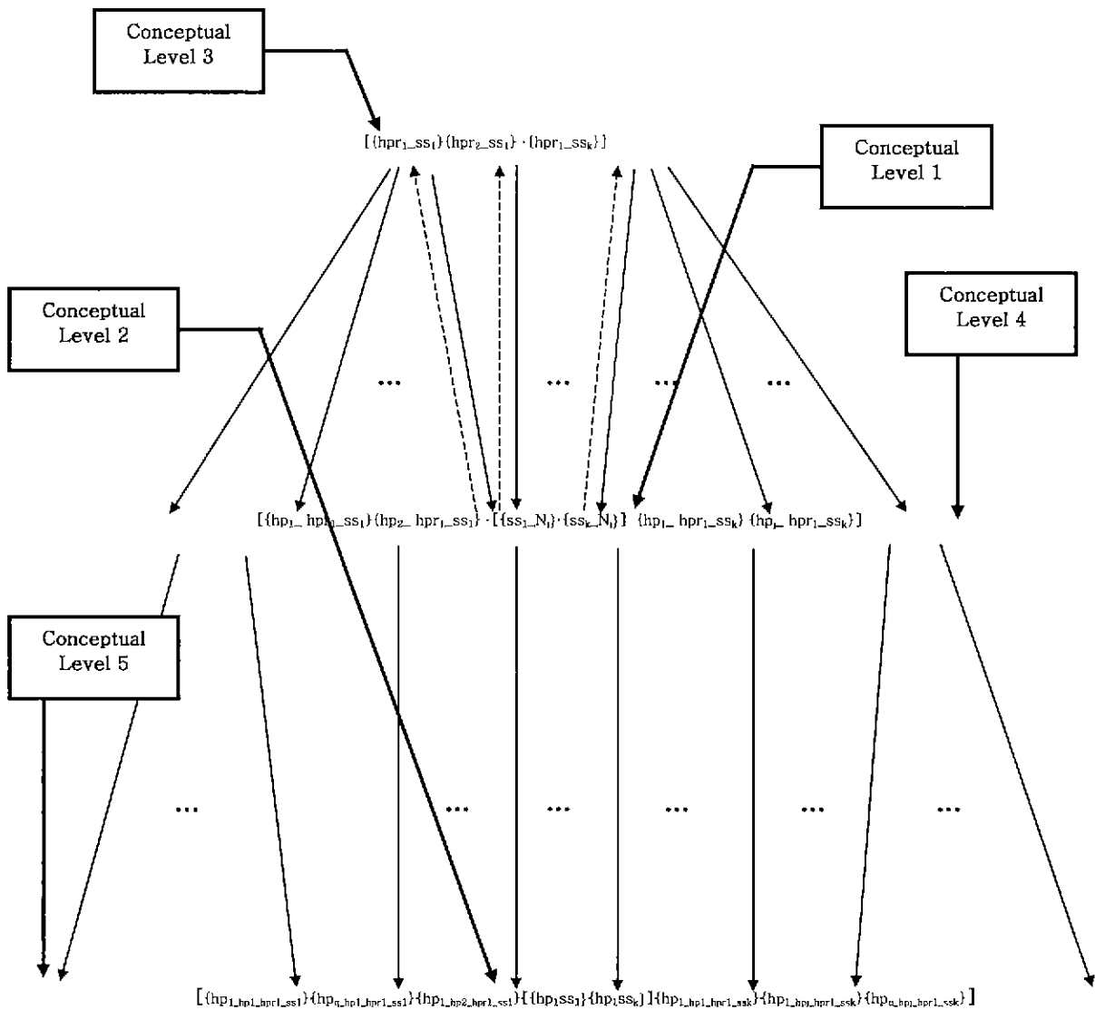
[그림 2] 통계 정보가 존재하지 않는 명사쌍 \langle N_i \rightarrow N_j \rangle 의 N_i 에 대한 개념레벨 적용
