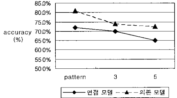
[그림 5] 창의 크기에 따른 Lauer모델의 정확률
