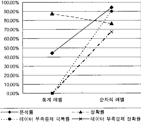
[그림 4] 순차적인 개념 레벨에서 분석률과 정확률
