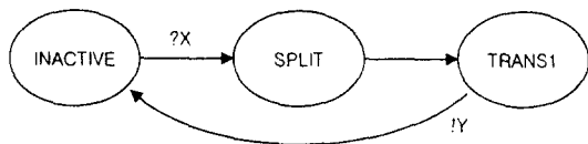
그림 3 State diagram of Route model
