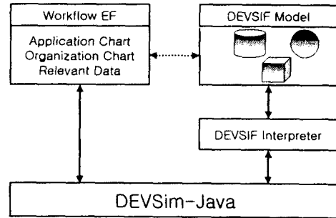
그림 4 Workflow 시물레이션 구조도
