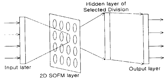
그림 1. 신경 회로의 구조
