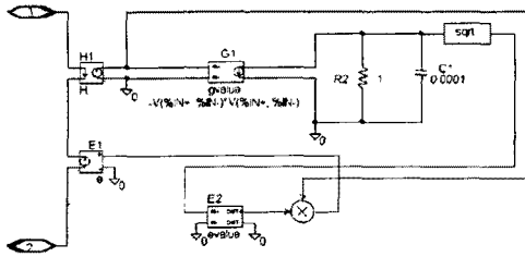
그림 1 PSPICE 램프 모델
