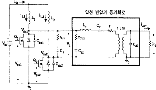
그림 10 압전 변압기를 이용한 Push-pull 인버터
