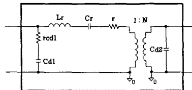
그림 9 압전 변압기 등가 회로
