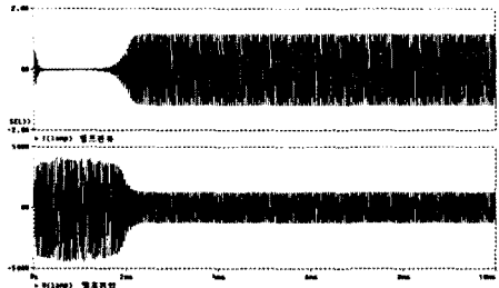
그림 6 CCFL 전류 및 전압 시뮬레이션 파형
