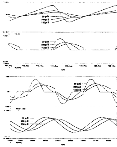
그림 14 L_1, L_2 가변시 인버터 각 단의 시뮬레이션 파형
