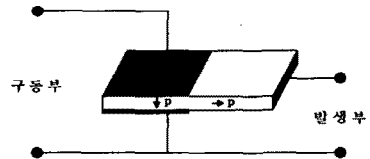
그림 7 압전 변압기
