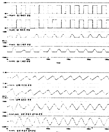
그림 11 Push-pull 인버터의 각 단 시뮬레이션 파형
