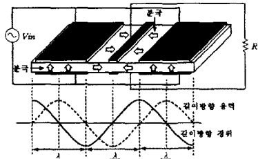
그림 8. 3차 길이방향 진동모드에서 동작하는 압전 변압기
