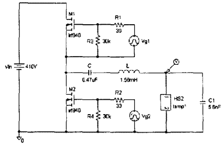
그림 5 전자 안정기의 시뮬레이션 회로
