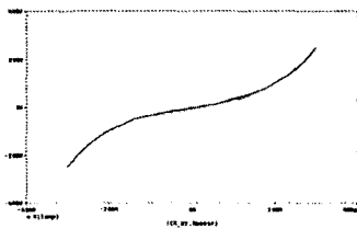
그림 4 램프의 V-I 특성곡선
