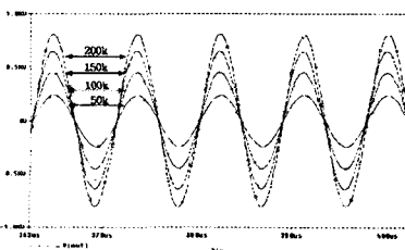
그림 12 부하저항 가변시 출력전압 파형
