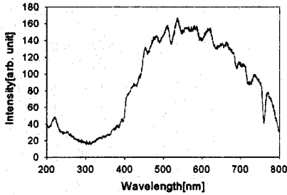
그림 5. 광파이버만을 통한 태양광의 스펙트럼 Fig. 5. Spectrum of sunlight through an optical fiber only
