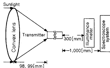
그림 4. 스펙트럼 및 조도 측정 Fig. 4. Schematic diagram of spectrum and illuminance measurements
