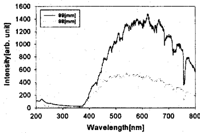
그림 6. 태양광 채광시스템을 통한 평균 스펙트럼 Fig. 6. Spectrum of sunlight through the sunlight collector system
