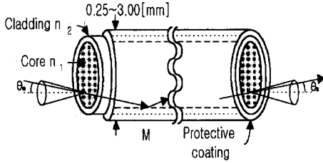
그림 3. 광파이버의 구조 Fig. 3. Structure of an optical fiber
