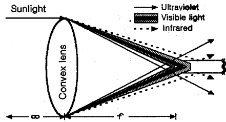
그림 2. 색수차를 이용한 태양광의 분리 Fig.2. Spectral zone selection utilizing chromatic aberration
