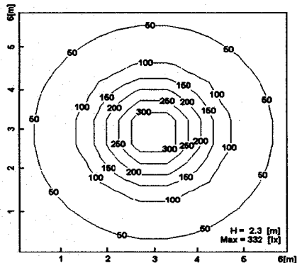
그림 7. 6기닥 한류용 광섬유 채광시스템에 대한 작업면의 조도분포 시뮬레이션 Fig. 7. Simulation of illuminance pattern on the work-plane for a sunlight collector system comprised of a bundle of six-core optical fibers
