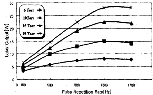
그림 3 펄스 반복율에 따른 레이저 출력 특성 Fig. 3 Laser output vs. pulse repetition rate
