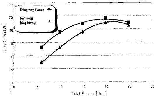
그림 5 가스 순환 여부에 따른 레이저 출력 특성 Fig. 5 Laser output vs. gas circulating with ring blower
