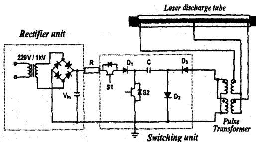
그림 2 고압 펄스 전원장치의 개략도 Fig. 2 Schematic diagram of high voltage pulsed power supply
