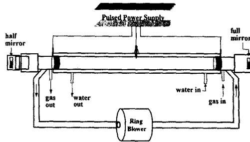
그림 1 저속 축류형 펄스 CO 2 레이저의 공진기 개략도
