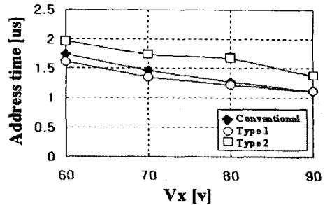
그림 7. V_x 변화에 따른 address time의 변화 Fig. 7 Variation of Address time as a parameter of V_x in address period
