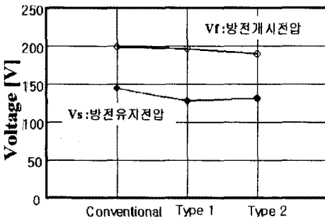
그림 5. Bus 전극 위치에 따른 방전전압 특성 Fig. 5 Characteristics of discharge voltage as a parameter of position of bus electrode.
