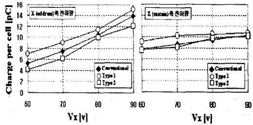
그림 6. V_x 변화에 따른 방전전하량의 변화 Fig. 6 Charge variation as a parameter of V_x in address period
