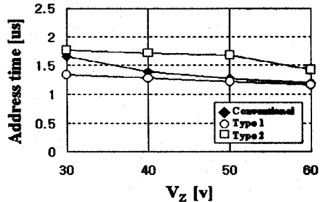
그림 11. V_z 변화에 따른 address time의 변화
