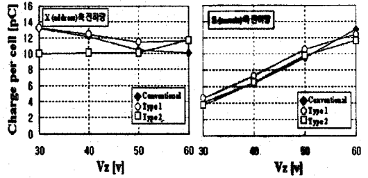
그림 10. V_z 변화에 따른 방전전하량의 변화
