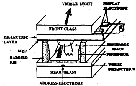
그림 1. ac PDP의 개략도
