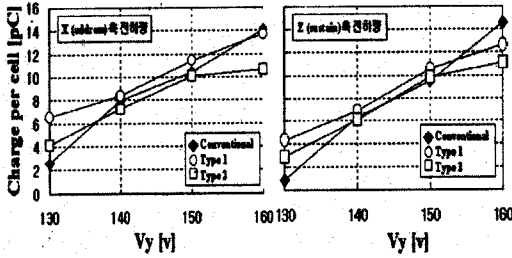
그림 8. V_y 변화에 따른 방전전하량의 변화
