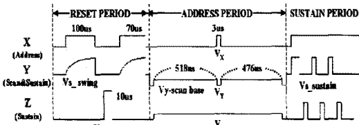
그림 4 구동 파형의 개략도 Fig. 4 Schematic diagram of driving waveform
