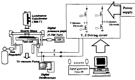
그림 3 방전특성 시험용 챔버의 개략도 Fig. 3 The schematic diagram of test chamber
