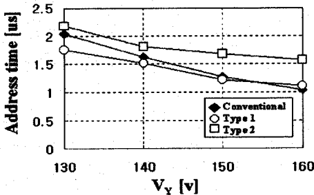
그림 9. V_y 변화에 따른 address time의 변화
