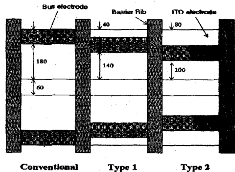
그림 2. 실험에 사용한 Bus 전극 위치에 따른 전극 구조
