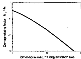
그림 1. Magnet 치수 비 r에 따른 반자장계수 N_d/4\pi
