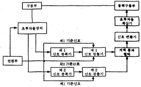
그림 4. 초투자율 측정 시스템의 블록도
