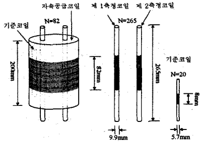
그림 2: 초투자율 측정장치
