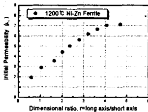
그림 5. Magnet 치수 비 r에 따른 하소온도에 따른 Ni-Zn Ferrite 분말의 초투자율
