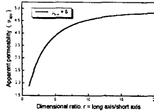
그림 6. Magnet 치수 비 r에 따른 가시투자율
