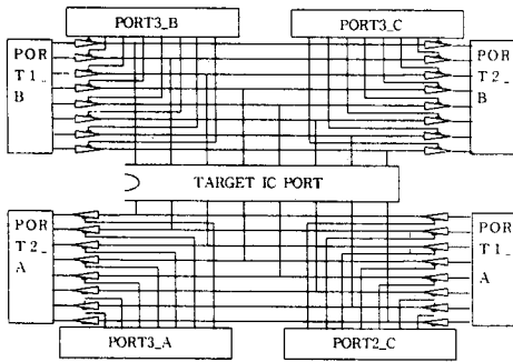
그림 3. TRI-STATE BUFFER BOARD 회로도
