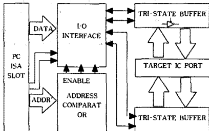
그림 1. 전체 BLOCK DIAGRAM
