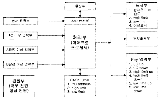
그림 1. 온·습도 계측 모듈의 구성도
