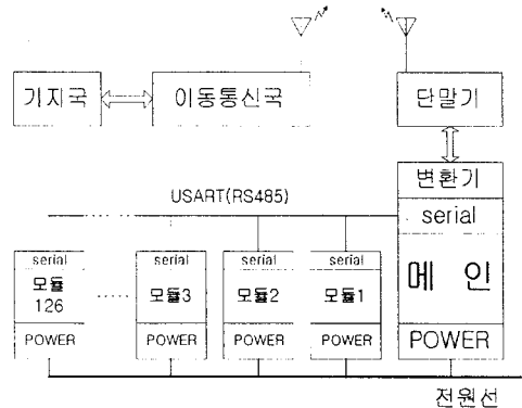
그림 2. 무인 원격감시 시스템의 전체 구성도
