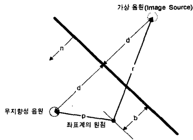
그림 1. 이미지 모델링의 원 음원과 가상 음원
