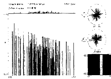
그림 4.e. 300,000개의 레이를 사용한 에코그램(극장)
