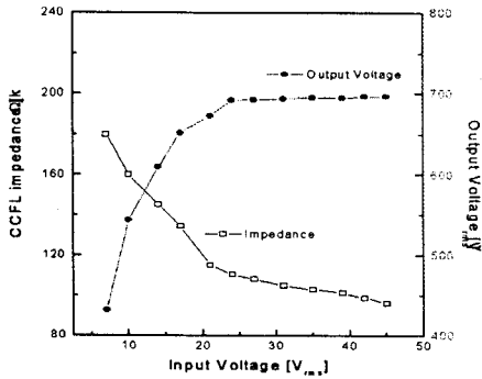
그림 6. 입력 전압에 따른 임피던스와 출력 전압
