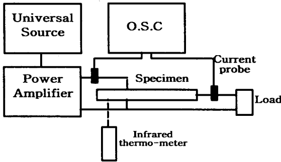
그림 2. 측정 시스템
