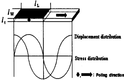
그림 1. λ진동모드형 압전 변압기의 구조와 변위 및 스트레스 분포
