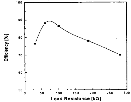
그림 4. 부하 저항에 따른 효율
