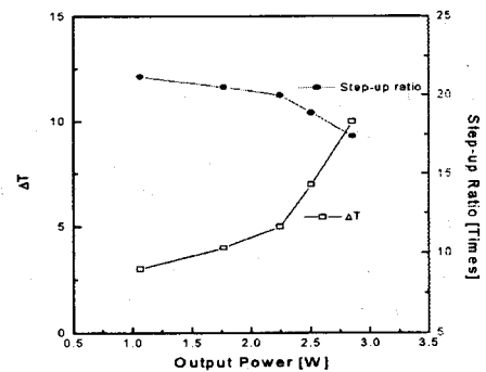
그림 5. 출력에 따른 승압비와 온도
