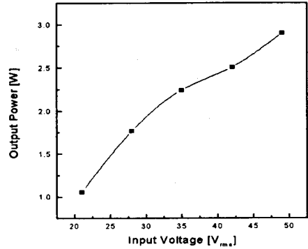
그림 3. 입력 전압에 따른 출력
