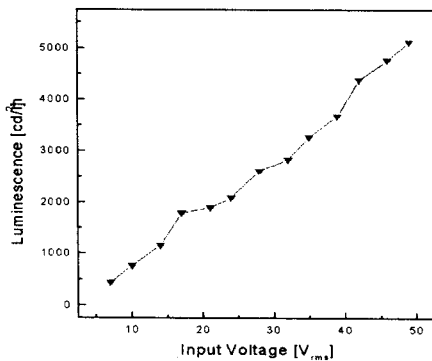
그림 7. 입력전압에 따른 휘도
