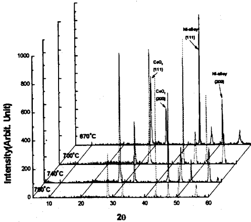
그림 2. 670~780°C에서 증착한 CeO 2 의 XRD 결과
