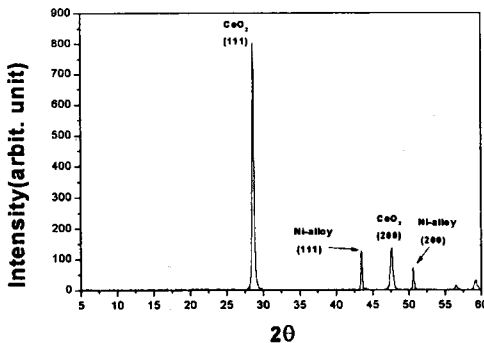
그림 4. 진공 상태에서 증착한 CeO 2 의 XRD 결과.
