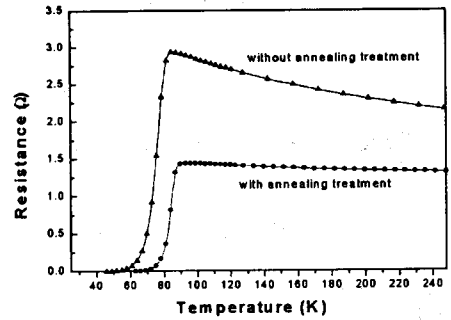
그림 5. 후열처리의 유무에 의한 임계온도의 변화
