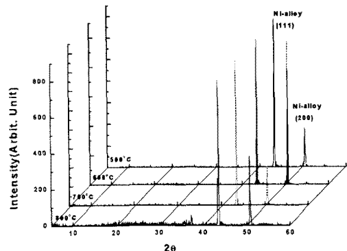
그림 1. 온도에 따른 Hastelloy의 XRD 분석 결과
