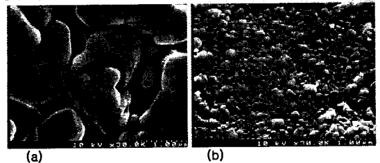
그림 6. (a) BTO위에 증착된 YBCO, (b) CeO 2 위에 증착된 YBCO의 SEM 결과
