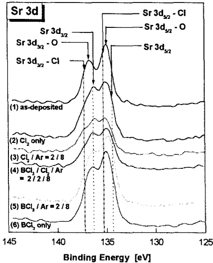
그림 3(b) BCl 3 /(Cl 2 +Ar) 가스비에 따라 식각된 BST 박막 표면에서의 Sr 3d XPS narrow scan spectra
