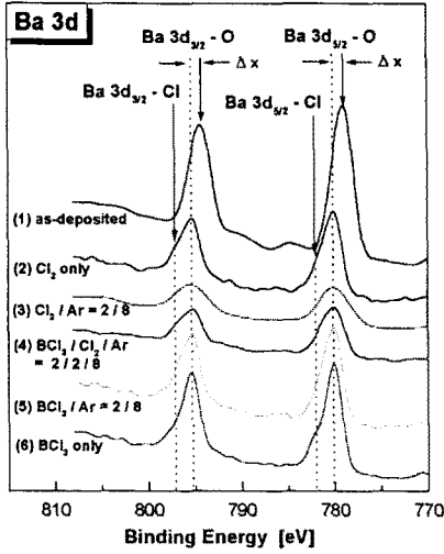
그림 3(a) BCl 3 /(Cl 2 +Ar) 가스비에 따라 식각된 BST 박막 표면에서의 Ba 3d XPS narrow scan spectra.
