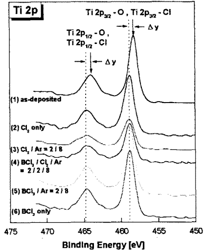
그림 3(c) BCl 3 /(Cl 2 +Ar) 가스비에 따라 식각된 BST 박막 표면에서의 Ti 2p XPS narrow scan spectra
