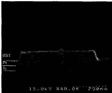
그림 4. BCl_3/Cl_2/Ar = 0.5/2/8 으로 식각된 BST 박막의 SEM 단면 사진.
