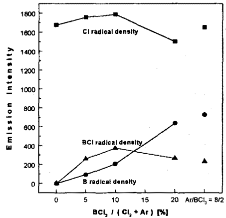
그림 2 Cl 2 /Ar 플라즈마에 BCl 3 가스첨가에 따른 상대적인 Cl, BCl and B의 라디칼 밀도.
