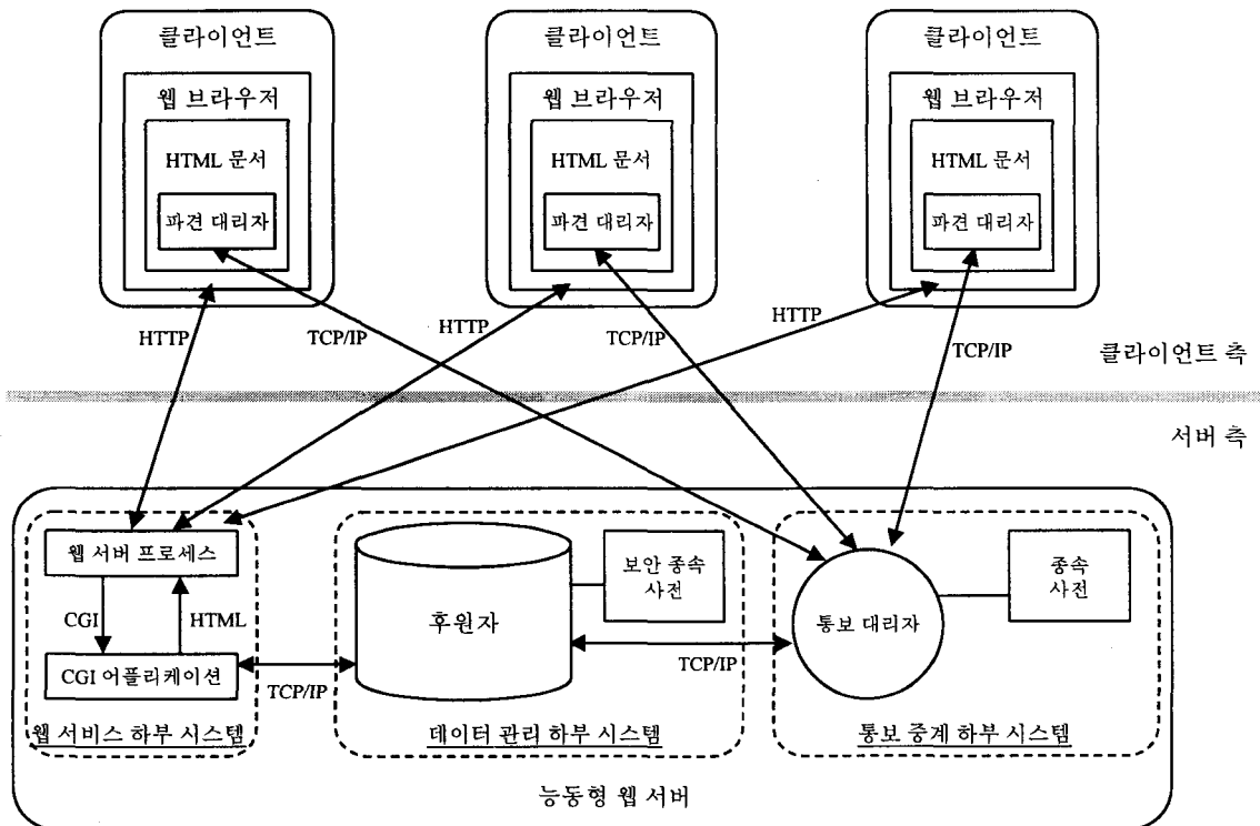
[그림 1] 능동형 웹 서버의 기본 구조도.
