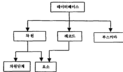
<그림 3-1> MDIS 메타데이터 스키마의 계층 구조
